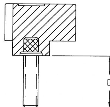
THREADED STUD
